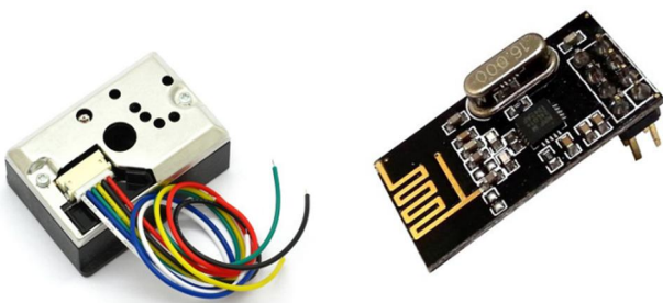
Hình 3. Cảm biến nồng độ bụi Sharp GP2Y1010AU0F và module RF NRF24L01
