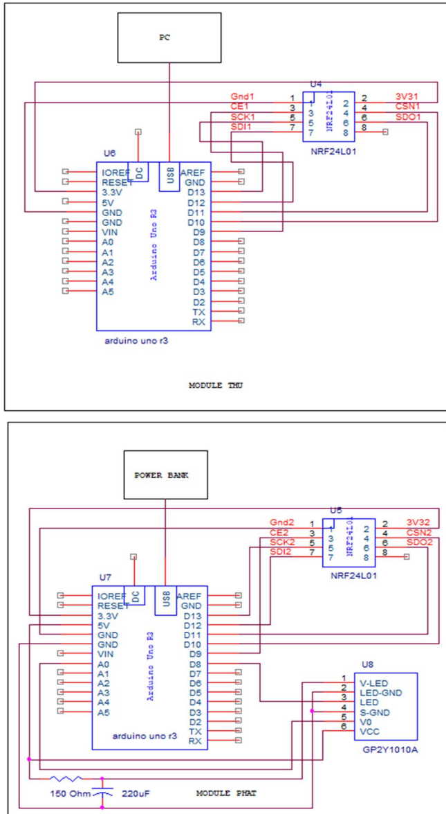
Hình 2. Mạch nguyên lý của hệ thống
