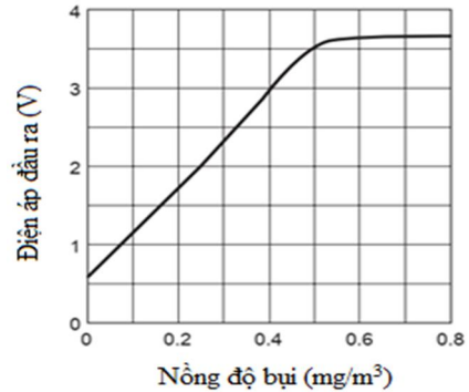
Hình 4. Biểu đồ tham khảo nhà sản xuất đưa ra về mối liên hệ giữa điện áp đầu ra và nồng độ bụi trên cảm biến Sharp GP2Y1010AU0F [1]
